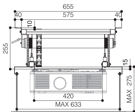
Punti di ancoraggio per proiettore
