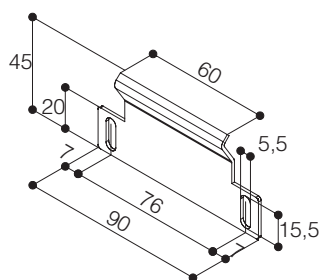
STAFFA DI ANCORAGGIO A PARETE
