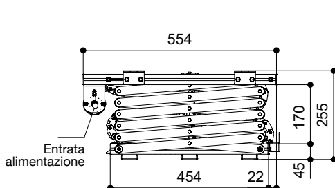
2.2.a - vista laterale
