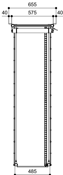
2.3.b - vista posteriore
