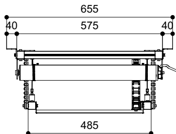
2.2.b - vista posteriore
