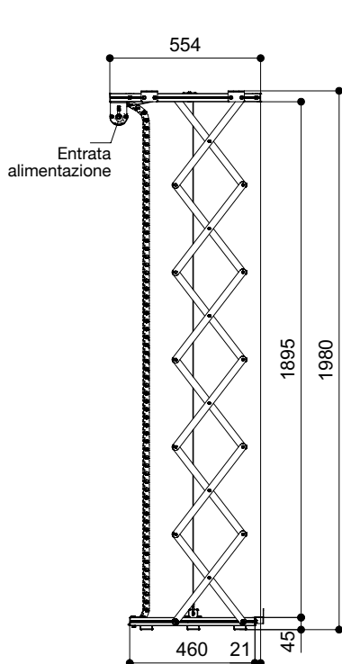
2.3.a - vista laterale
