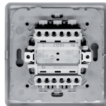
Motore/Motor Moteur/Motor/Motor 230v - 50Hz ⏏ T Giallo/verde Green/Yellow Vert/Jaune Grün/Gelb Verde/amarillo ① N Blu Blue Bleu Blau Azul ② L Marrone Brown Marron Braun Marron ③ Nero Black Noir Schwarz Negro 3 x 1.5 mm 2
